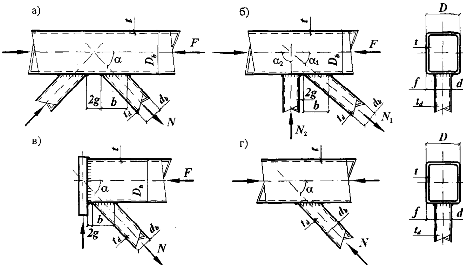
a – К-образный при треугольной решетке; b – то же, при раскосной решетке; c – опорный; z – У-образный
