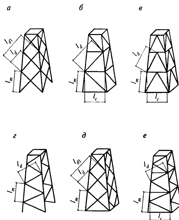
a, б, в — с совмещенными в смежных гранях узлами; г, д — с не совмещенными в смежных гранях узлами; е — с частично совмещенными в смежных гранях узлами
