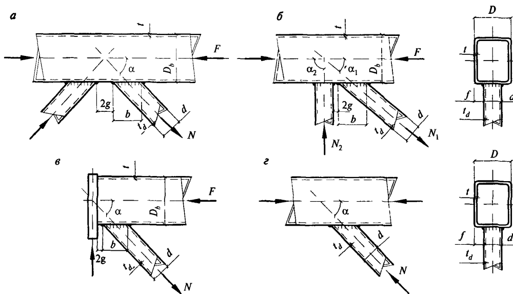
a — К-образный при треугольной решетке; b — то же, при раскосной решетке; c — опорный; d — У-образный
